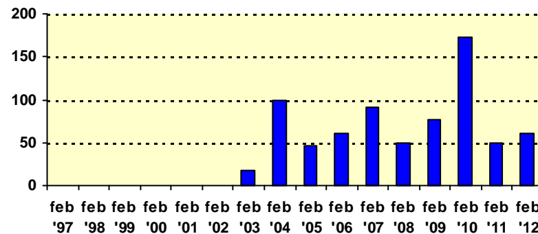
Precipitazioni mm
