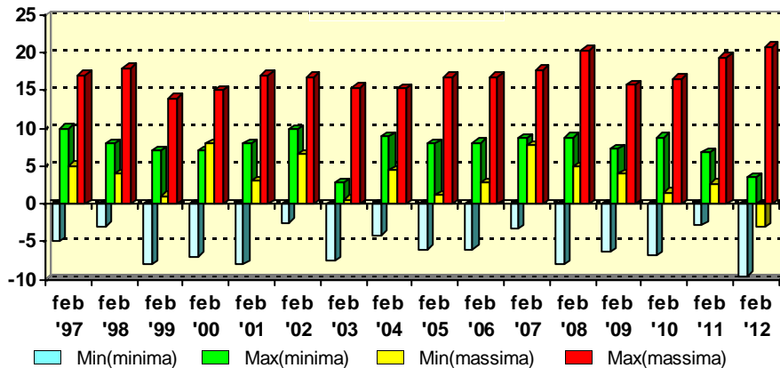
Estremi termici
