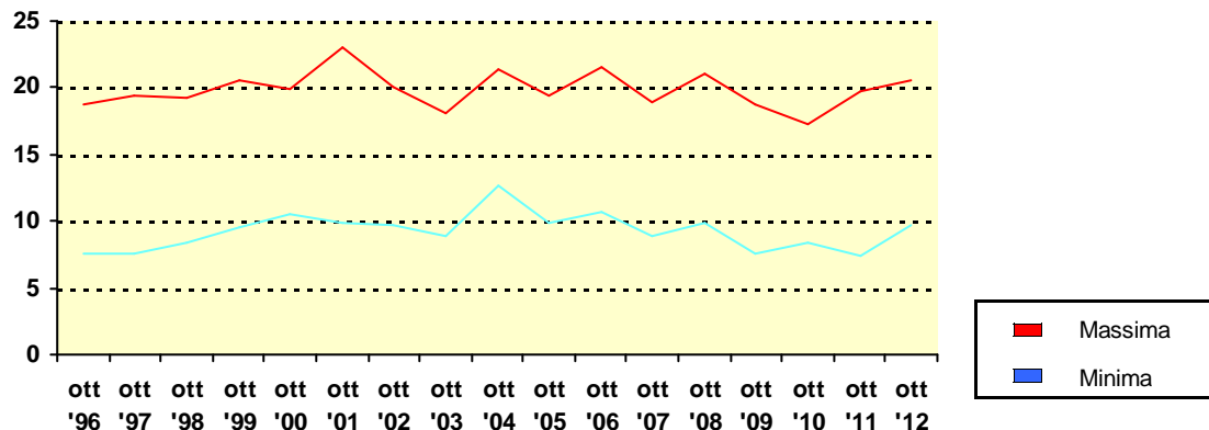
Temperatura °C
