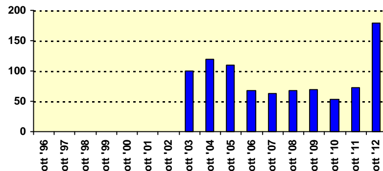
Precipitazioni mm
