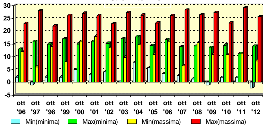
Estremi termici
