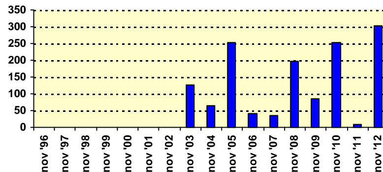
Precipitazioni mm
