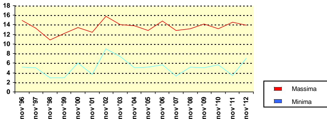
Estremi termici
